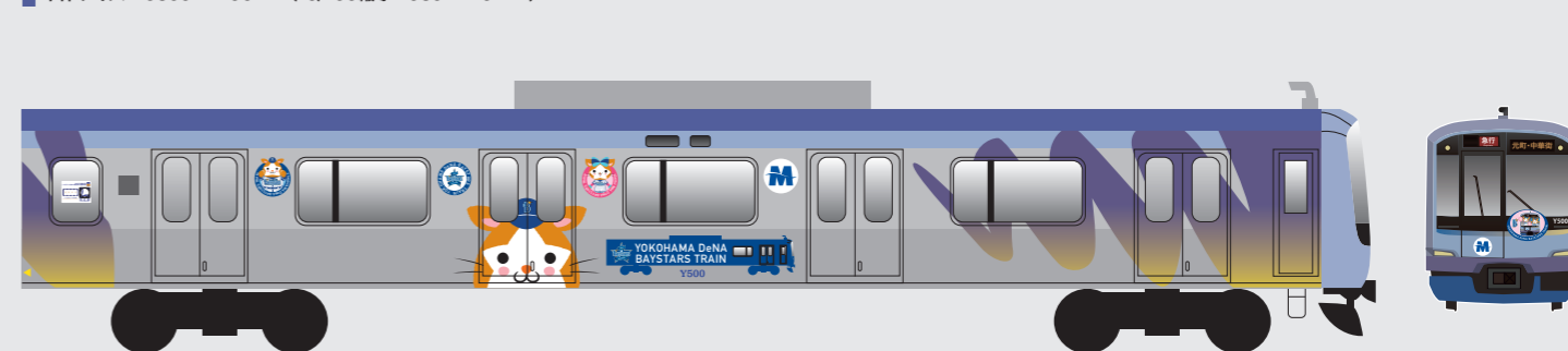
Y500系 元町・中華街方面先頭8号車 車体サイズ:19800×2290mm (10/100縮小 1980×229mm)
