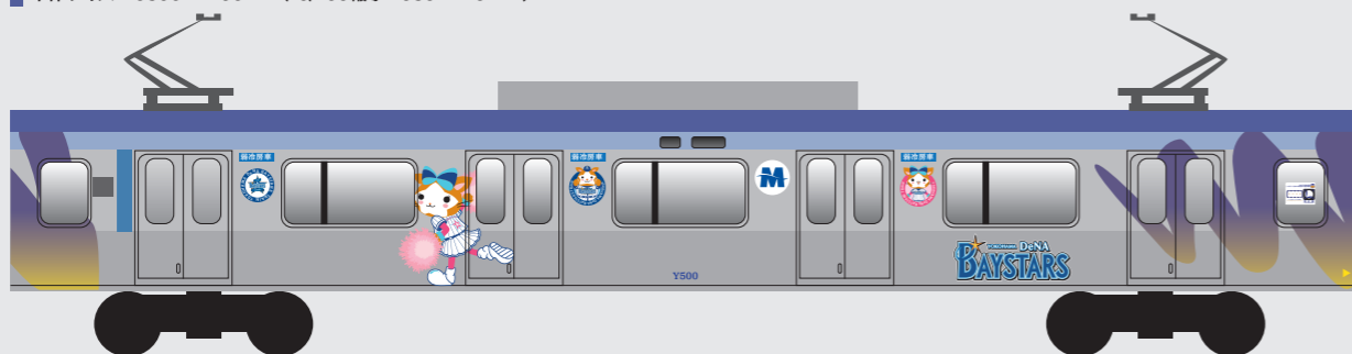
Y500系 7号車 車体サイズ:19500×2290mm (10/100縮小 1950×229mm)
