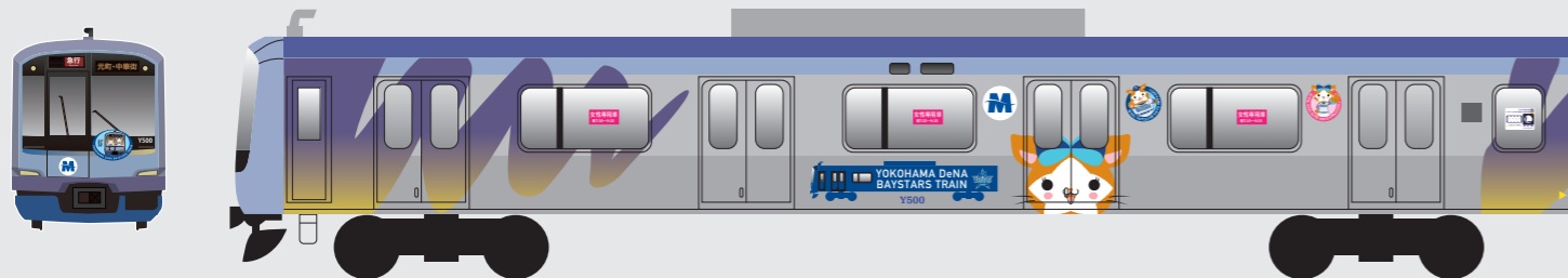
Y500系 横浜方面先頭1号車 車体サイズ:19800×2290mm (10/100縮小 1980×229mm)
