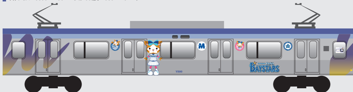
Y500系 3号車 車体サイズ:19500×2290mm (10/100縮小 1950×229mm)
