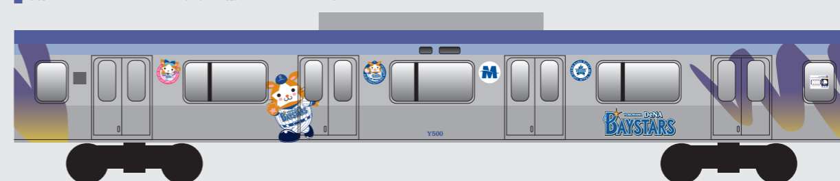
Y500系 6号車 車体サイズ:19500×2290mm (10/100縮小 1950×229mm)
