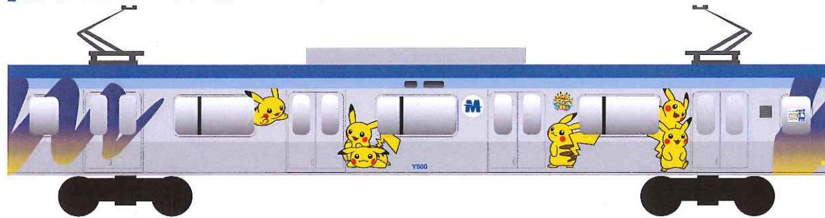
Y500系 6号車 車体サイズ:19500×2290mm(10/100縮小 1950×229mm)
